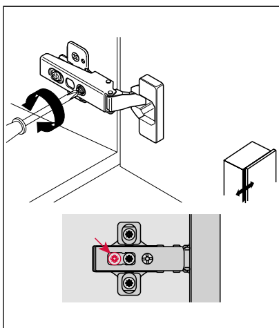
Seitenverstellung: -1,5 bis 4,5 mm
