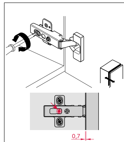
Tiefenverstellung: -0,5 bis +2,8 mm
