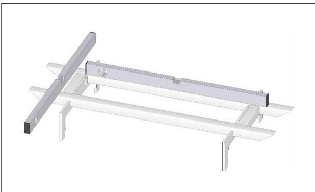
Gestell ausrichten Align the frame
