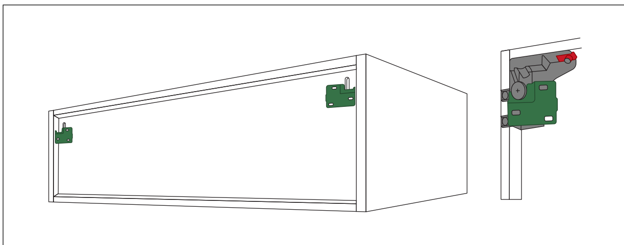
Wandhängebeschläge, Einstellung vom Hersteller Assembly manufacturer
