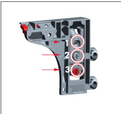
Vertikale Einstellung (13mm): vertical adjustments (13mm):
