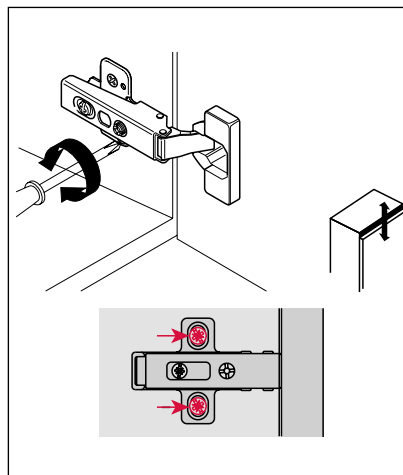
Höhenverstellung: \pm 2 mm
