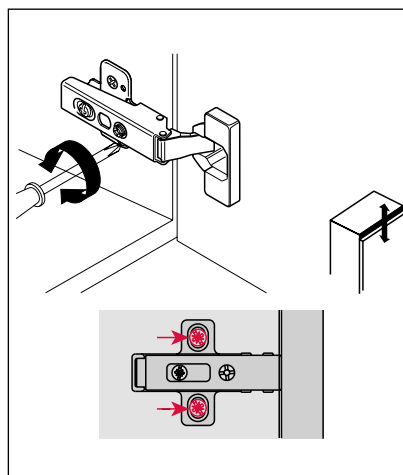
Höhenverstellung: ±2 mm
