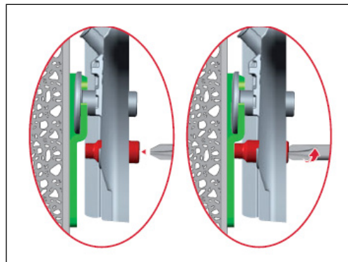
Bitte stoppen Sie das drehen, wenn der rote Einsatz an die Platte stößt Stop screwing the red bolt when it touches the plate
