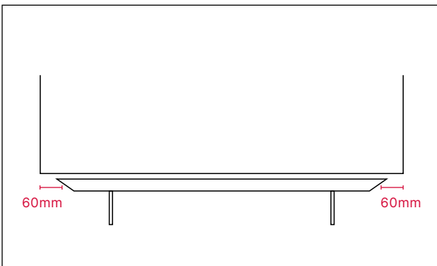
Korpus links und rechts 60mm vermitteln Position the carcass left and right with a distance of 60mm
